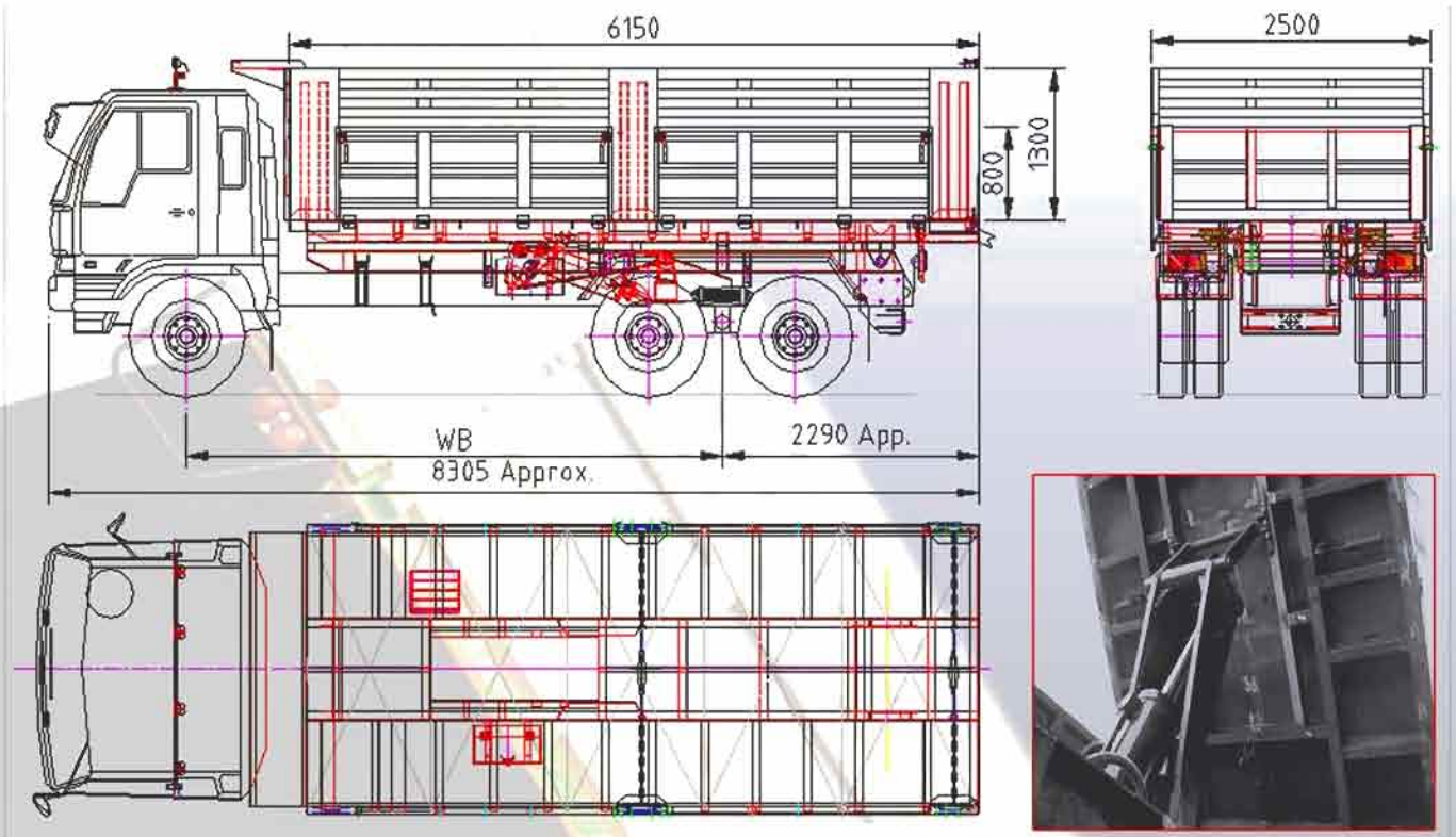
แบบมาตรฐานที่ติดตั้งกับรถยนต์บรรทุก 10 ล้อ
